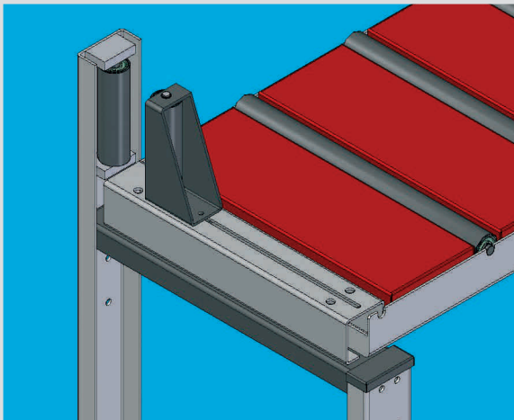
Rodillo vertical para la guía del material Vertical roll for material clamping
