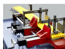
» Dispositivo de corte en paquete mecánico
